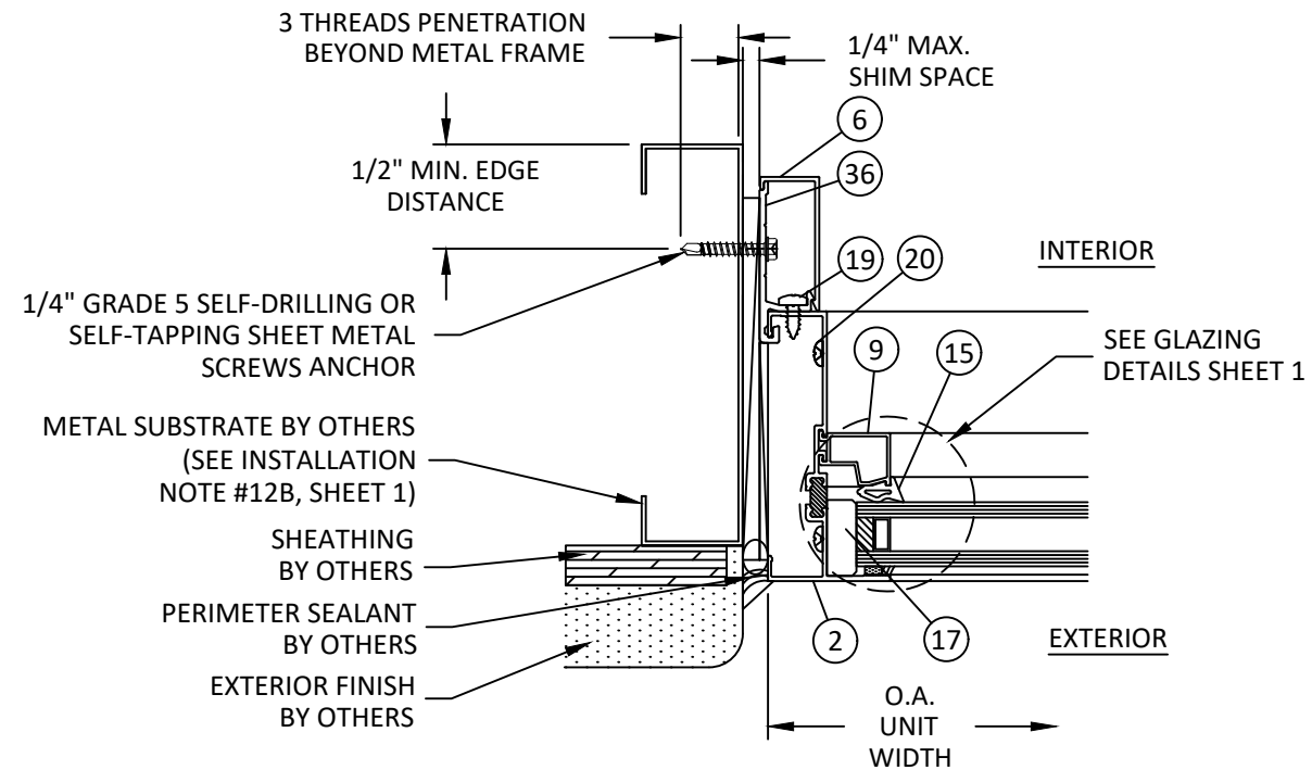
G 6 HORIZONTAL SECTION JAMB - STEEL STUD CLIP ANCHOR
