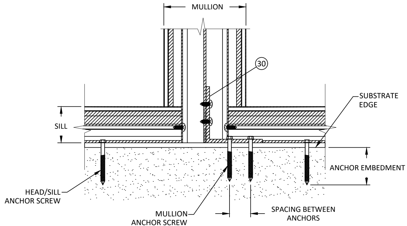
N 8 MULLION LONGITUDINAL SECTION
