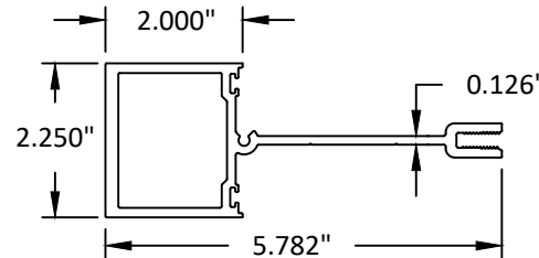
5 STACKING MULLION (TUBULAR) 6063-T5
